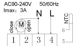
Vízmelegítési kapcsolási rajz
