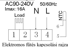
Elektromos fűtés kapcsolási rajza
